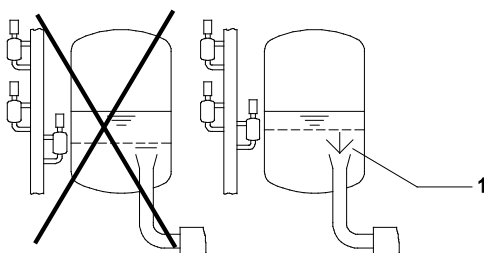
Abb. 11: Anordnung Niveauüberwachung
