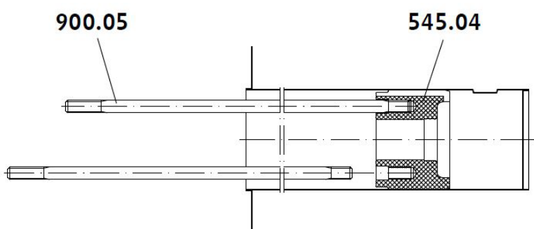
Abb. 16: Demontage des Kohlelagers – CAMh
