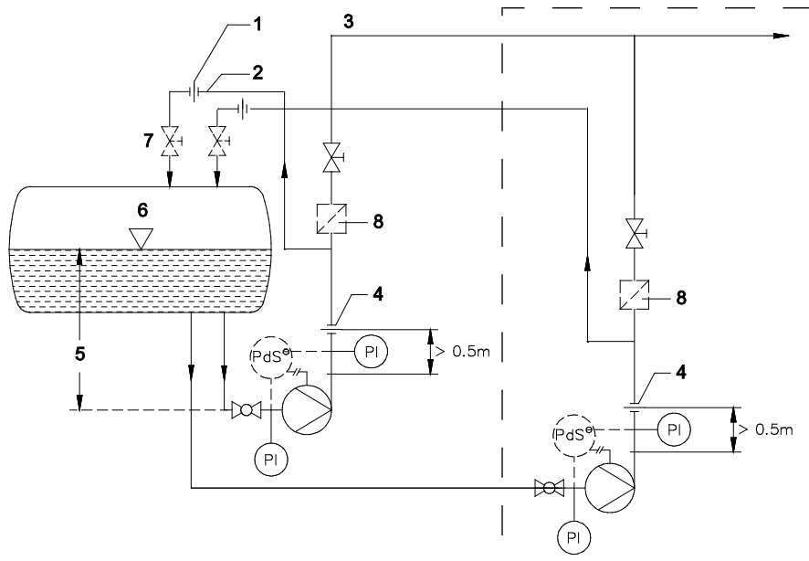
Abb. 14: Automatische Entgasung (Einzelpumpe-Parallelpumpen)
