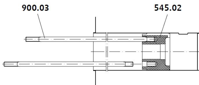
Abb. 15: Demontage des Kohlelagers – CAM
