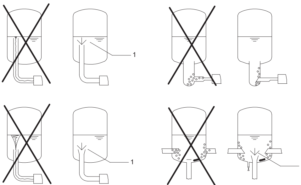
Abb. 9: Anordnung Rotationsbrecher am Tankauslauf
