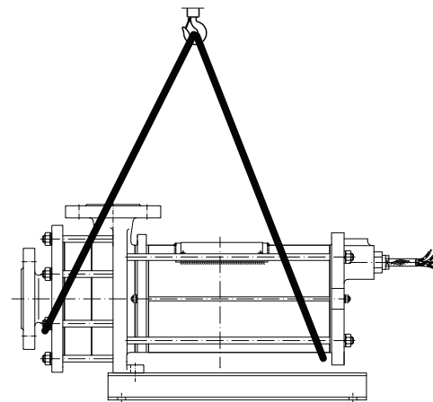
Abb. 6: Hebezeug befestigen an Pumpenaggregat mit Grundplatte
