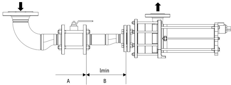
Abb. 8: Zulaufleitung und Beruhigungsstrecke
