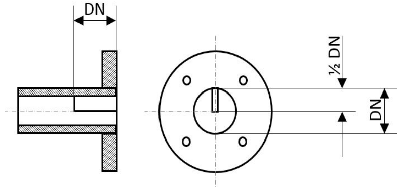
Abb. 7: Rohrleitung mit Drallbrecher
