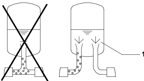
Abb. 12: Anordnung Parallelbetrieb
