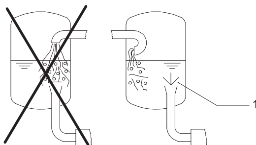
Abb. 10: Anordnung Tankeinlauf/Tankauslauf
